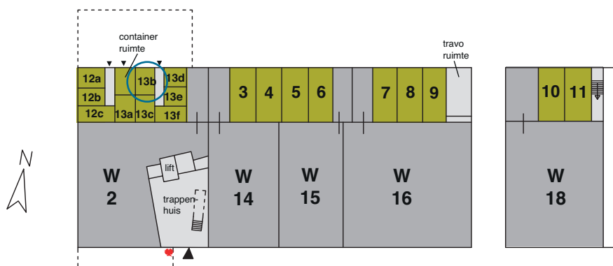
Begane grond
